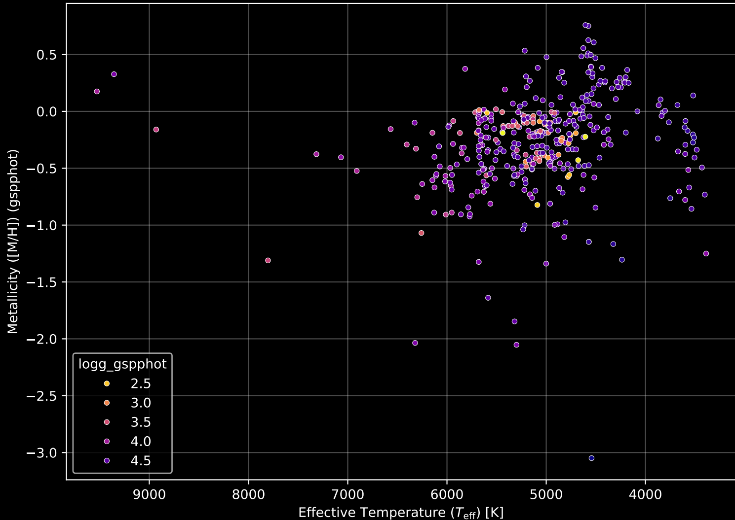
APOGEE DR17 Field: [ORPHAN-5] Stellar Population Parameters (n= 391)
